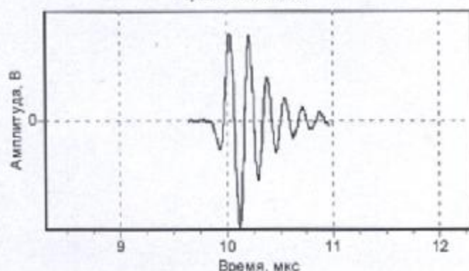
Форма эхосигнала
