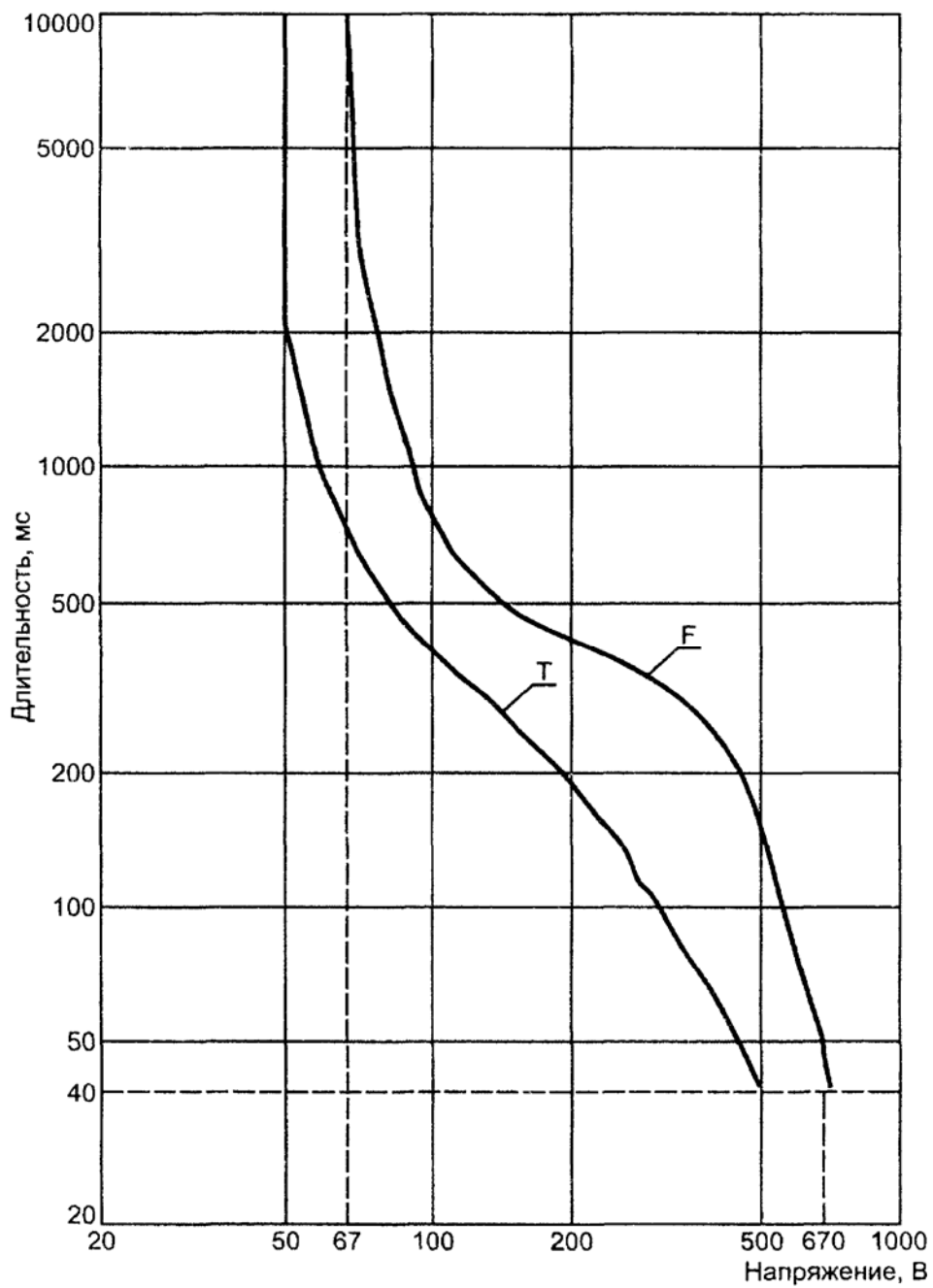
Рисунок 44А — Зависимость напряжения замыкания (кривая F ) и ожидаемого напряжения прикосновения (кривая T ) от максимальной длительности замыкания на землю на стороне выше 1 кВ
