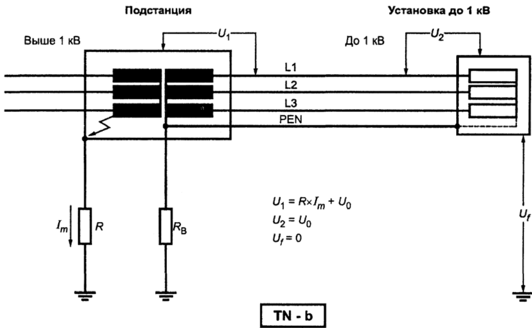
Рисунок 44В — TN-системы
