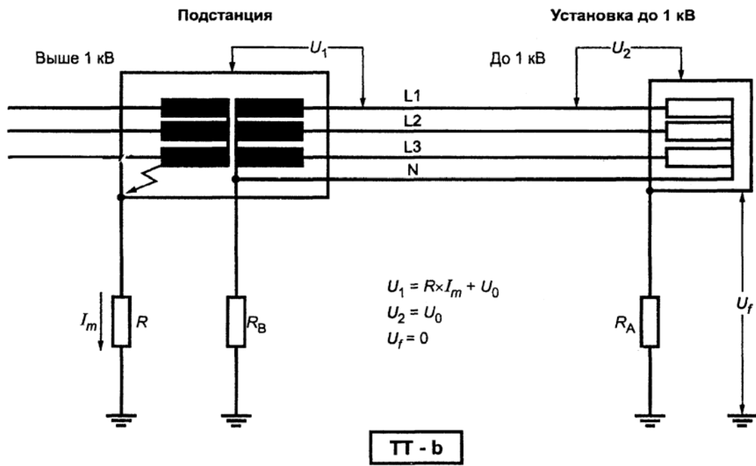
Рисунок 44С — ТТ- системы
