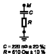
Рисунок 6 — Схема эквивалента руки (см. 6.2.5)
