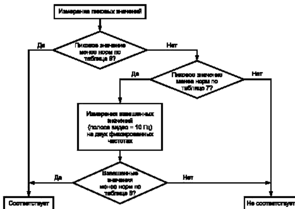
Рисунок 5 — Алгоритм принятия решения по результатам измерений излучаемых ИРП в полосе частот от 1 до 18 ГГц ПНМБ ВЧ устройств класса А и класса В, группы 2, работающих на частотах свыше 400 МГц
