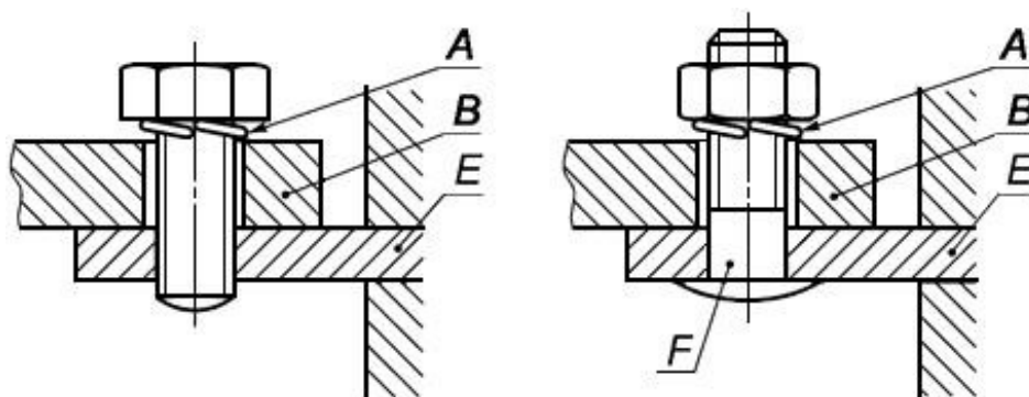
Рисунок IC.4 - Примеры выводов для кабельных наконечников
