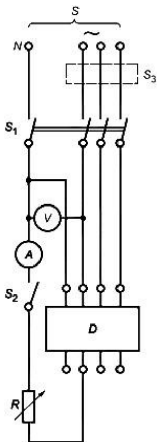
Рисунок 4а - Испытательная цепь для проверки: рабочих характеристик; механизма свободного расцепления; поведения в случае исчезновения напряжения сети для АВДТ, функционально зависящих от напряжения сети
