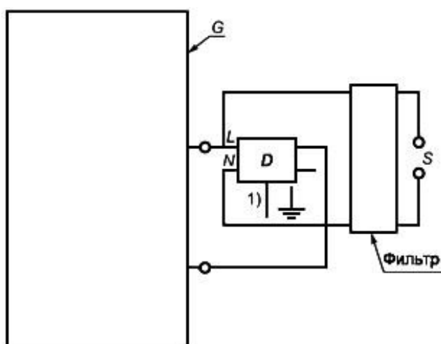
Рисунок 26 - Схема испытания АВДТ звенящей волной
