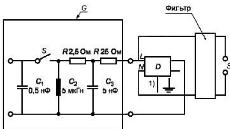
Рисунок 24 - Испытательная цепь для испытания АВДТ звенящей волной
