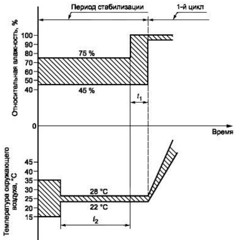
Рисунок 20 - Период стабилизации для испытаний на надежность
