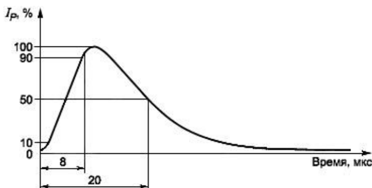
Рисунок 25 - Звенящая волна 8/20 мкс
