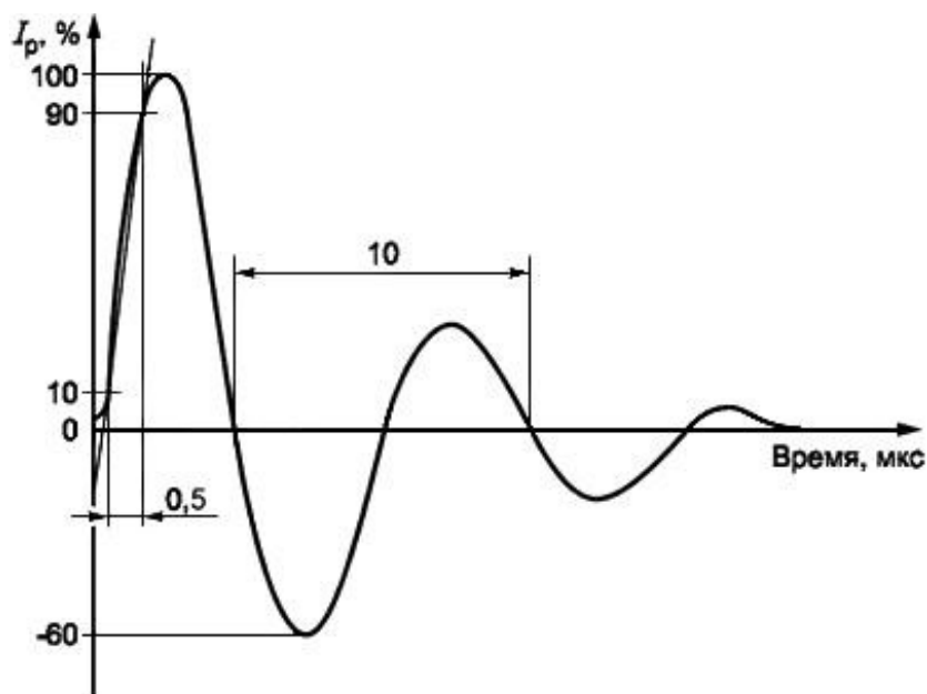
Рисунок 23 - Ток звенящей волны 0,5 мкс/100 кГц
