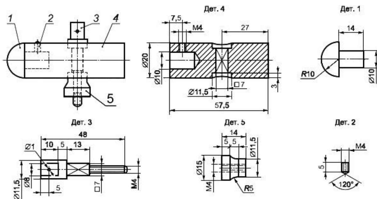
Рисунок 13 - Ударный элемент маятникового устройства для испытаний на механический удар
