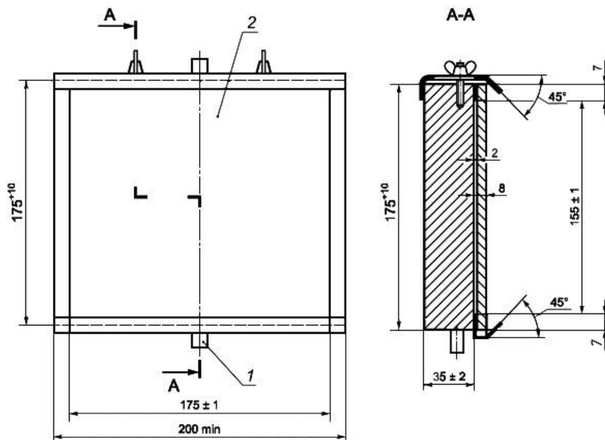
Рисунок 14 - Монтажное основание устройства для испытаний на механический удар
