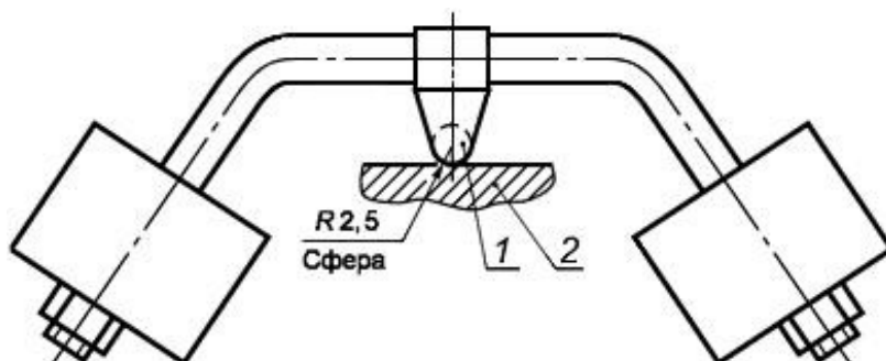
Рисунок 18 - Устройство для испытания давлением шарика
