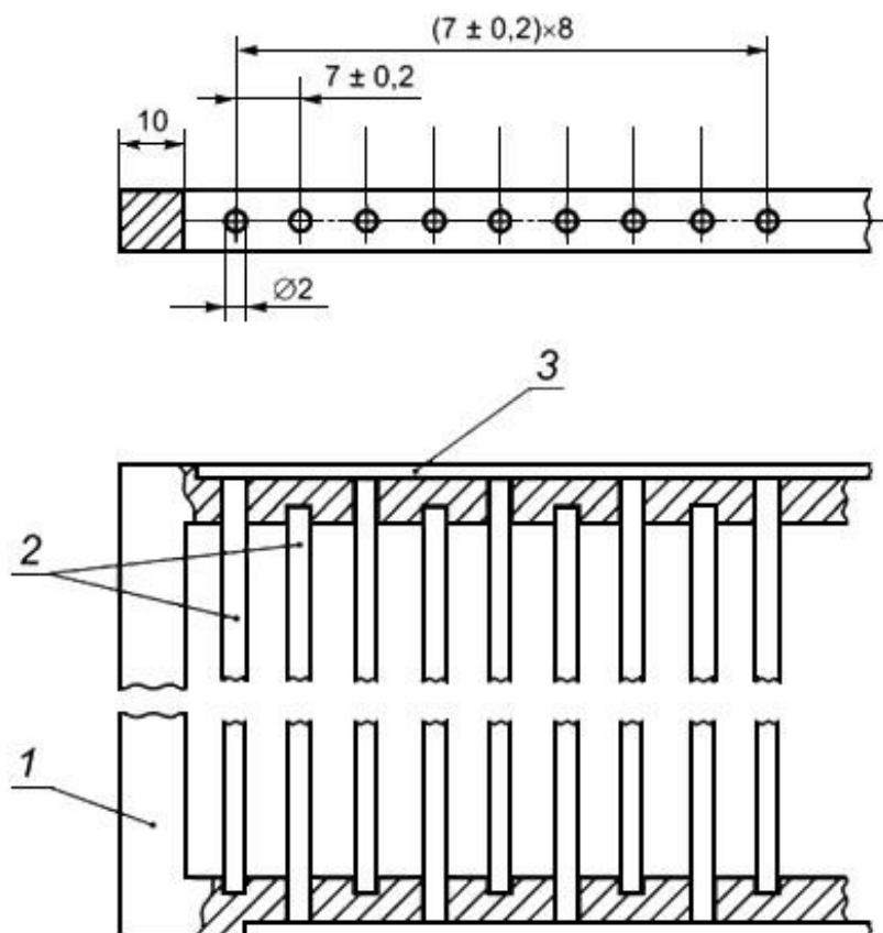
Рисунок С.2 - Сетка
