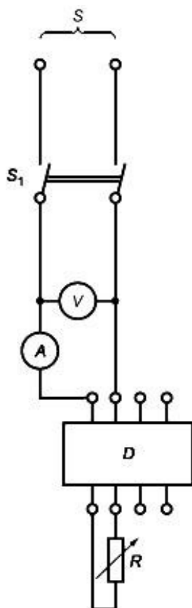
Рисунок 19 - Испытательная цепь для проверки предельных значений перегрузки по току в случае однофазной нагрузки трех- или четырехполюсного АВДТ
