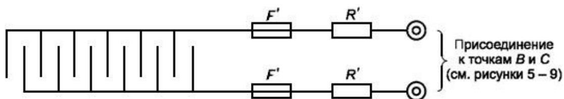
Рисунок С.3 - Цепь сетки
