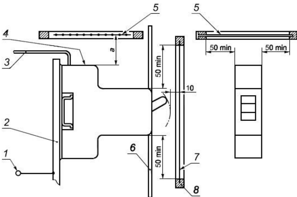
Рисунок С.1 - Испытательное устройство
