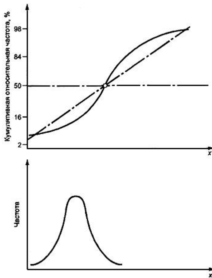
Рисунок 4 - Кумулятивная функция распределения (вверху) и функция плотности распределения с большой кривизной (внизу)
