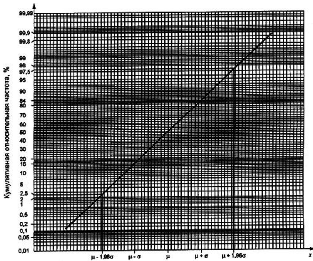
Рисунок 1 - Бумага для нормальных вероятностных графиков
