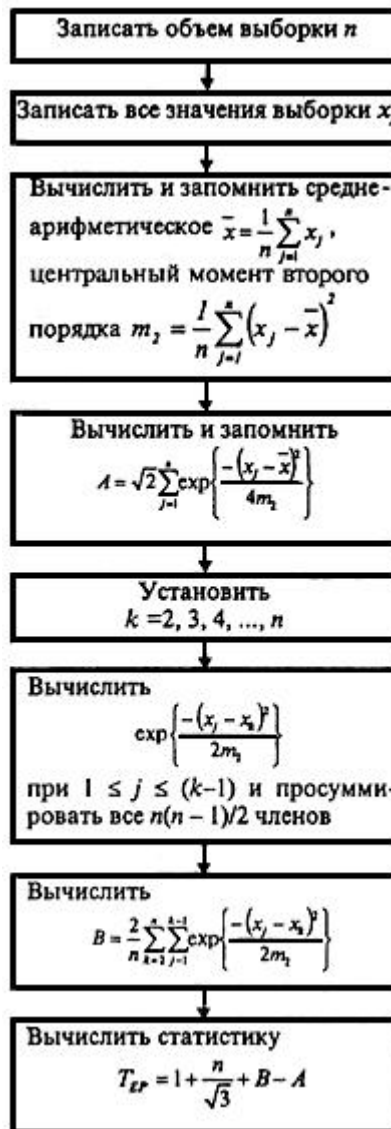
Рисунок 8 - Алгоритм вычисления статистики критерия Эппса-Палли
