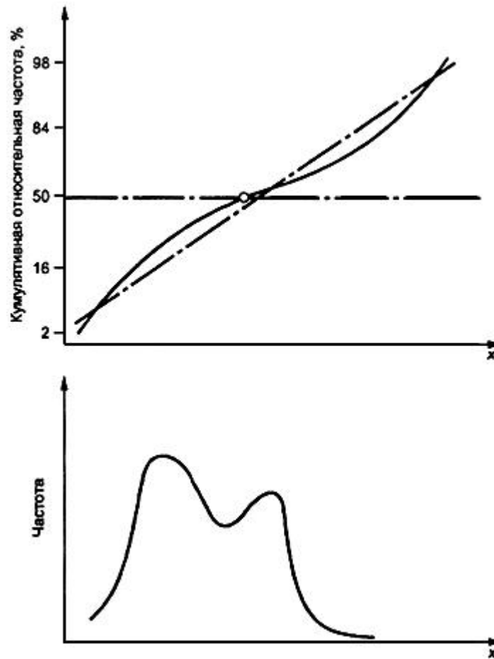
Рисунок 7 - Функции, полученные наложением двух различных кумулятивных функций распределения (вверху) и функций плотности распределения (внизу)
