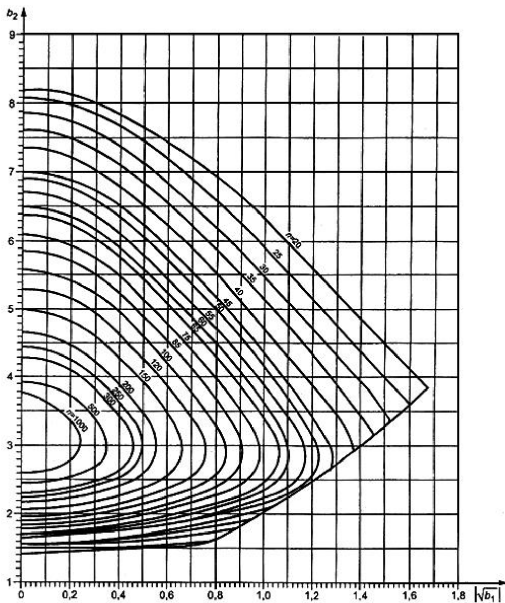
б) Кривые, выделяющие критическую область на уровне значимости \alpha = 0,01
