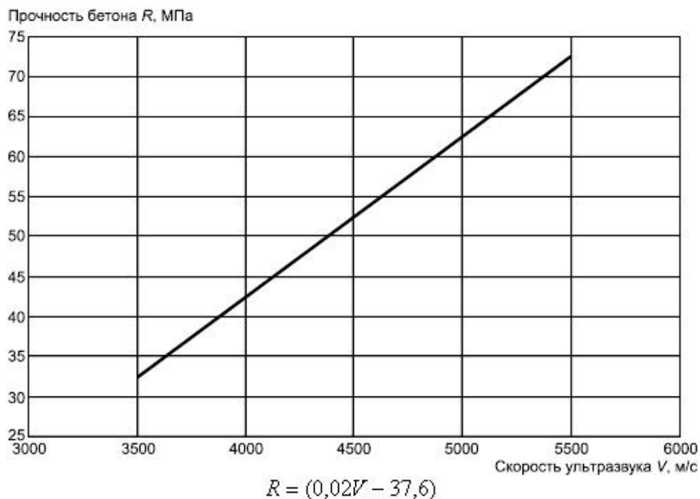
Рисунок Г.2 - Универсальная градуировочная зависимость, построенная по результатам испытаний конструкций из бетона проектных классов В35-В60
