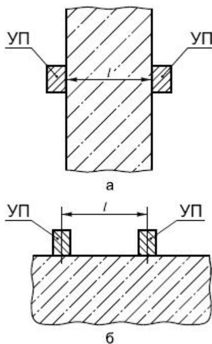
Рисунок А.1 - Схемы испытания бетона ультразвуковым методом
