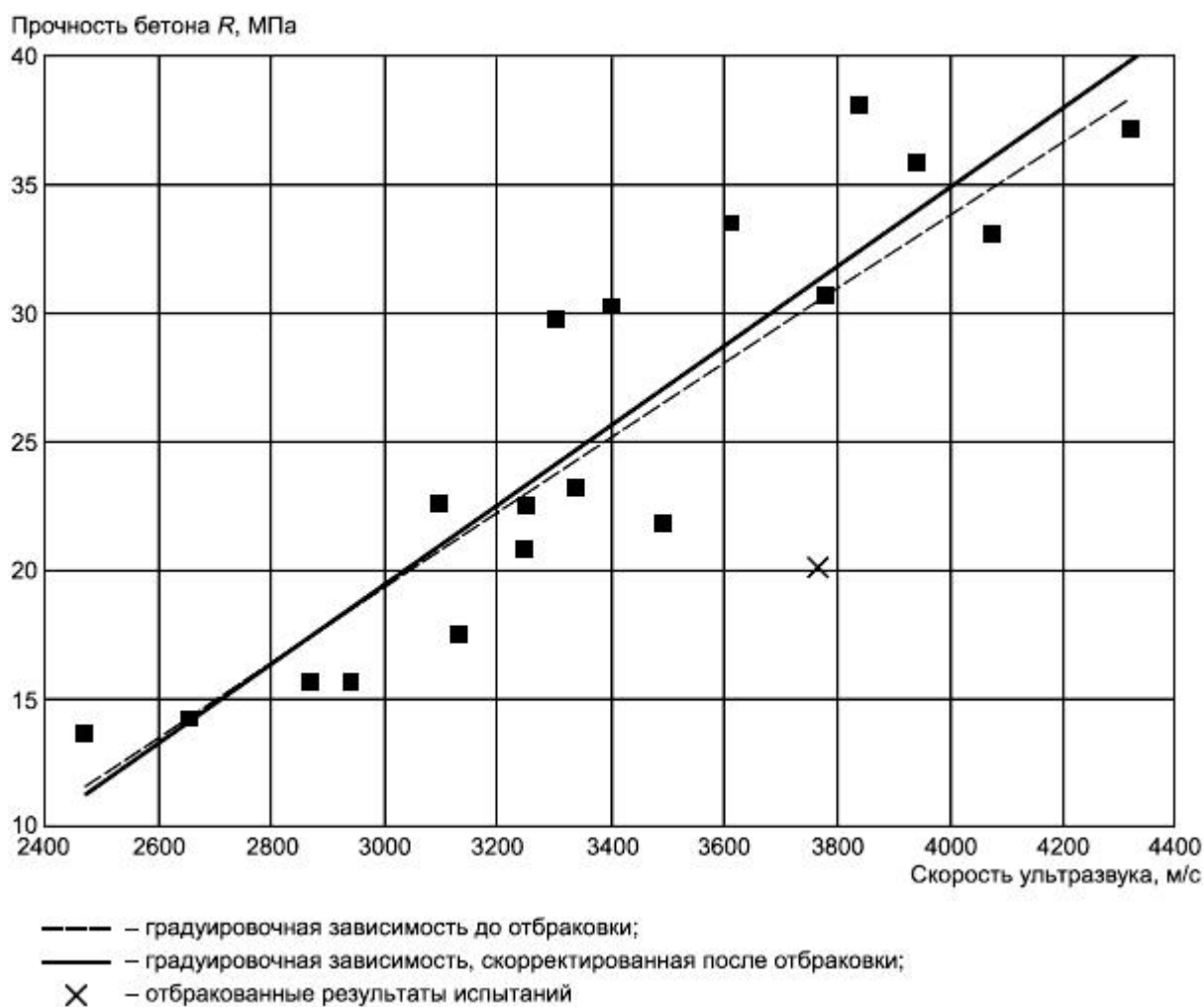
Рисунок В.1 - Градуировочная зависимость
