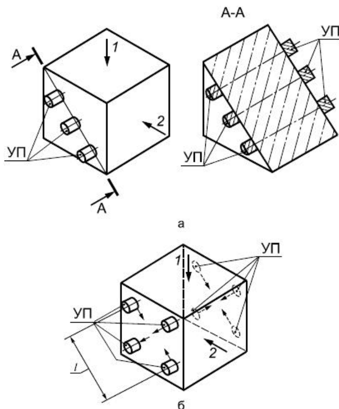
а - схема испытания образцов-кубов способом сквозного прозвучивания; б - схема испытания образцов-кубов способом поверхностного прозвучивания; УП - ультразвуковые преобразователи; - база прозвучивания; 1 - направление формования; 2 - направление испытания при сжатии
