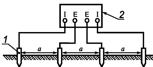
1 - электрод, 2 - прибор с клеммами: I - токовыми; E - измерительными; a - расстояния между электродами (см. формулу (А.1))
