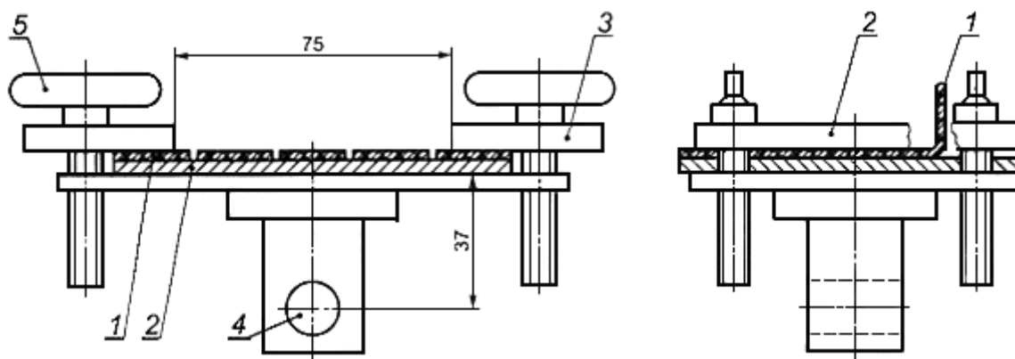
1 - защитное покрытие; 2 - металлическая подложка (образец из трубы); 3 - струбцина; 4 - отверстие для крепления струбцины к захвату разрывной машины; 5 - крепежный винт Рисунок А.2 - Струбцина для крепления образцов
