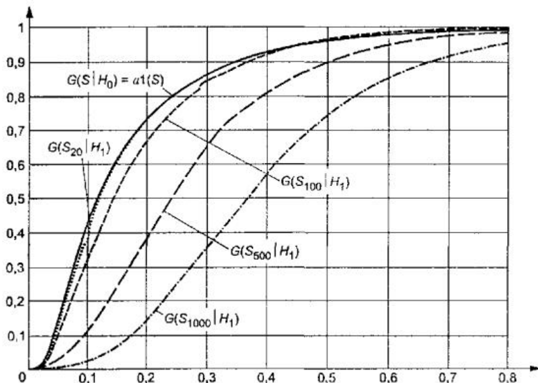
Рисунок 7 - Зависимость от n распределений G(S_n^{1/2}H_1) статистики S_\omega Крамера - Мизеса - Смирнова при простой гипотезе ( H_0 - нормальное распределение, H_1 - логистическое): n = 20, 100, 500, 1000
