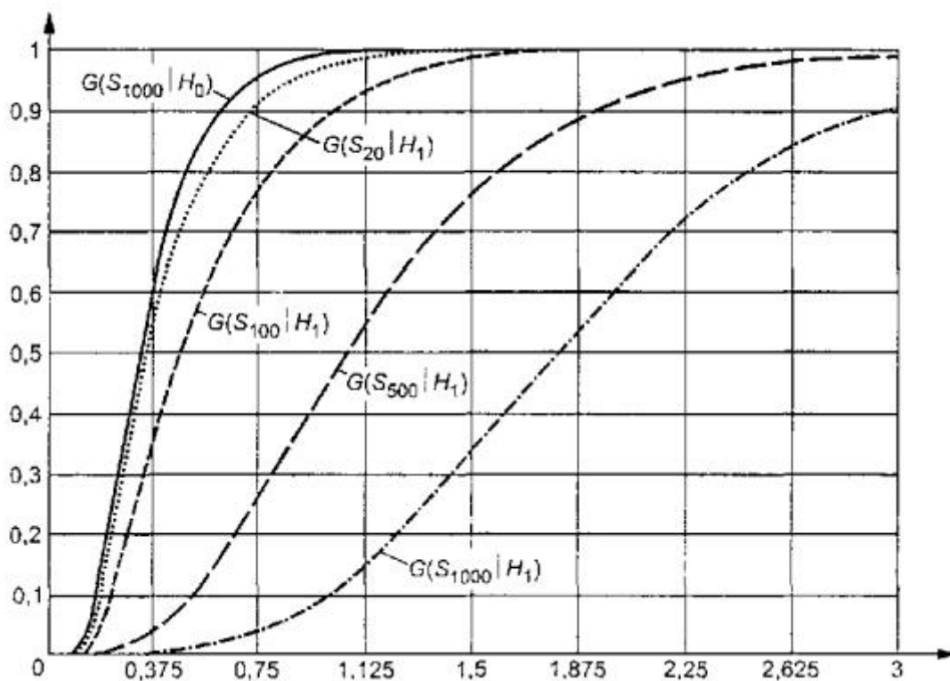
Рисунок 19 - Зависимость от n распределений G(S_n^{1/2} | H_1) статистики S_\Omega Андерсона - Дарлинга при сложной гипотезе ( H_0 - нормальное распределение; H_1 - логистическое; ОМП): n = 20, 100, 500, 1000
