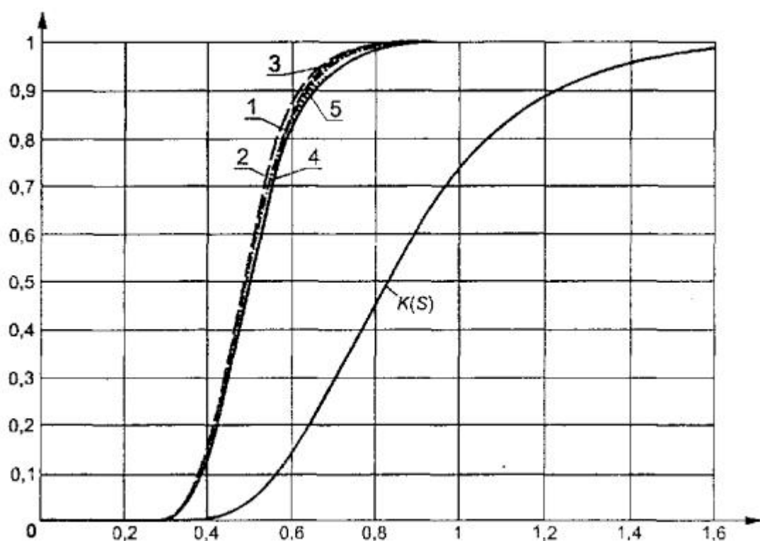
Рисунок 11 - Распределения G(S_n^{1/2}H_0) статистики Колмогорова S_K при оценивании двух параметров закона, соответствующего гипотезе H_0 , при использовании MD-оценок S_K . K(S) - функция распределения Колмогорова, предельная при простой гипотезе
