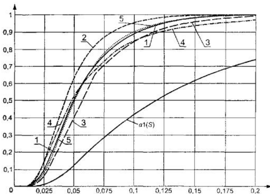
Рисунок 12 - Распределения G(S_n^{1/2}H_0) статистики S_w Крамера - Мизеса - Смирнова при оценивании двух параметров закона, соответствующего гипотезе H_0 , при использовании ОМП. a1(S) - функция распределения, предельная при простой гипотезе
