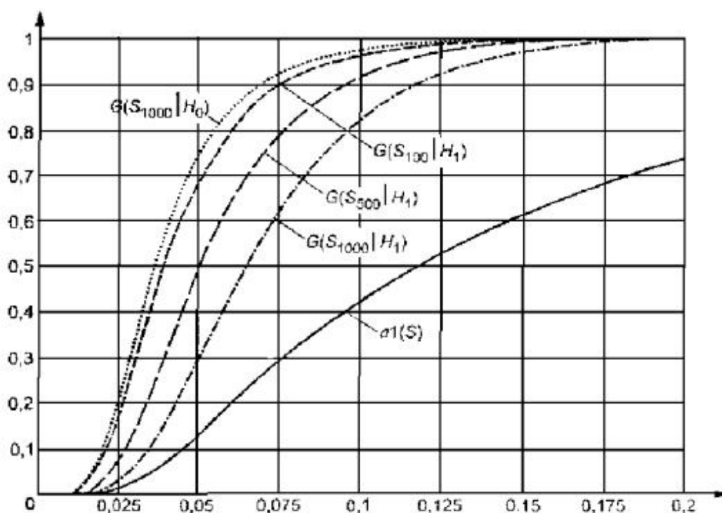
Рисунок 18 - Зависимость от n распределений G(S_n^{1/2} | H_1) статистики S_\omega Крамера - Мизеса - Смирнова при сложной гипотезе ( H_0 - нормальное распределение; H_1 - логистическое; MD-оценки S_\omega ): n = 100, 500, 1000
