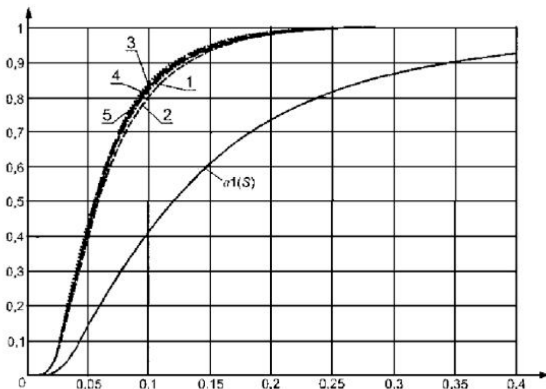
Рисунок 16 - Распределения G(S_n^{1/2}H_0) статистики S_{\omega} Крамера - Мизеса - Смирнова при оценивании масштабного параметра закона, соответствующего гипотезе H_0 , (1 - экспоненциального; 2 - полунормального; 3 - Рэлея; 4 - Максвелла; 5 - модуля 5-мерного нормального вектора), при использовании MD -оценок S_{\omega}
