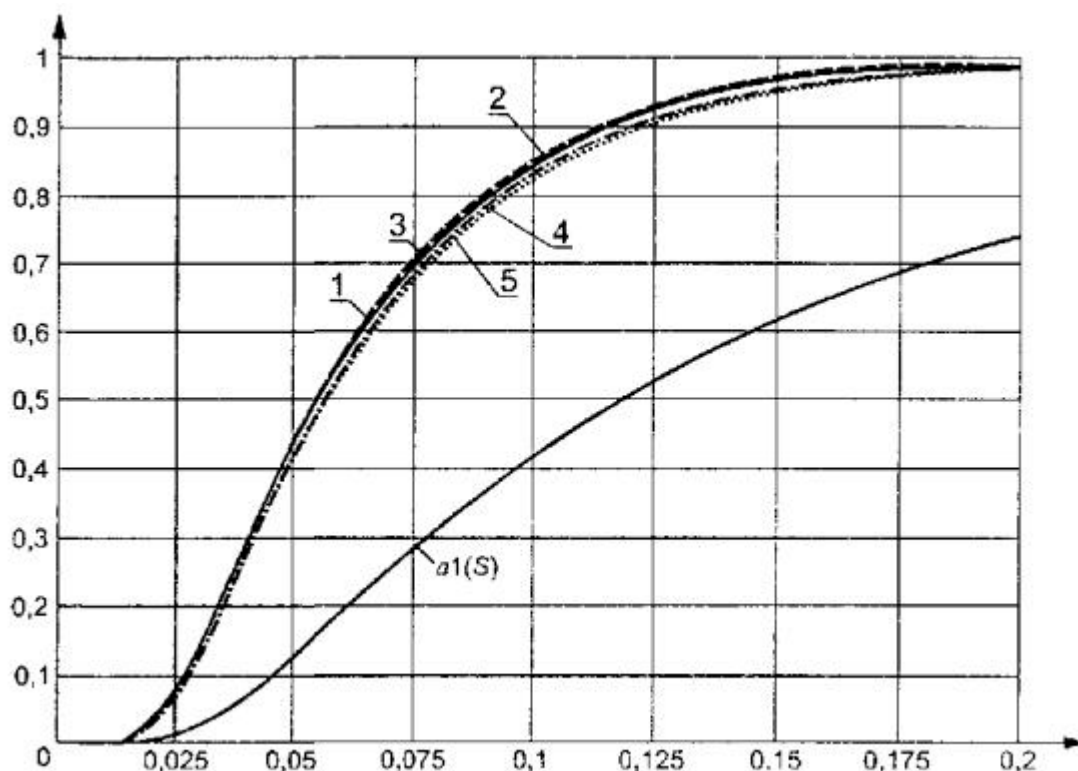
Рисунок 15 - Распределения G(S_n^{1/2}H_0) статистики S_0 Крамера - Мизеса - Смирнова при оценивании параметра сдвига, соответствующего гипотезе H_0 , при MD-оценках S_0
