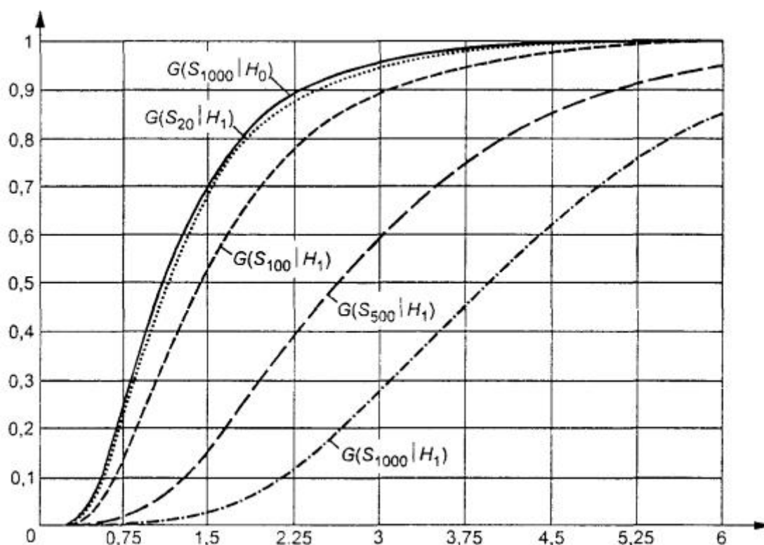
Рисунок 20 - Зависимость от n распределений G(S_n^{1/2} | H_1) статистики S_m Смирнова при сложной гипотезе ( H_0 - нормальное распределение; H_1 - логистическое; ОМП): n = 20, 100, 500, 1000
