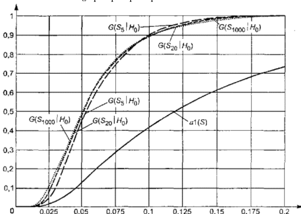
Рисунок 3 - Зависимость от n распределений G(S_n^{1/2}H_0) статистики S_\omega Крамера - Мизеса - Смирнова при сложной гипотезе ( H_0 - нормальное распределение, ОМП): n = 5, 20, 1000
