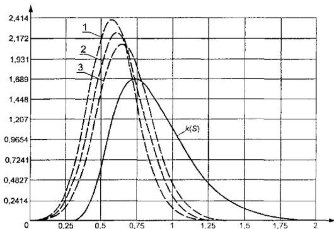
Рисунок 9 - Плотности распределения g(S_n^{1/2}H_0) статистики S_K при проверке сложной гипотезы ( H_0 - нормальный закон, оценивание сдвига с использованием 1 - MD-оценок S_K ; 2 - MD-оценок S_\omega ; 3 - ОМП). k(S) - плотность распределения Колмогорова
