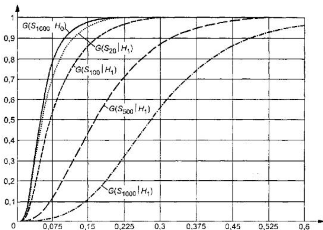
Рисунок 8 - Зависимость от n распределений G(S_n^{1/2}H_1) статистики S_0 Крамера - Мизеса - Смирнова при сложной гипотезе ( H_0 - нормальное распределение, H_1 - логистическое, ОМП): n = 20, 100, 500, 1000
