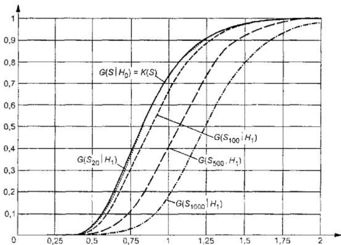
Рисунок 5 - Зависимость от n распределений G(S_n/2 | H_1) статистики S_K Колмогорова при простой гипотезе ( H_0 - нормальное распределение, H_1 - логистическое): n = 20, 100, 500, 1000
