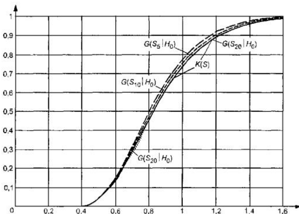
Рисунок 1 - Зависимость от n распределений G(S_n/2 H_0) статистики S_K Колмогорова при простой гипотезе ( H_0 - нормальное распределение): n = 5, 10, 20 . K(S) - функция предельного распределения Колмогорова
