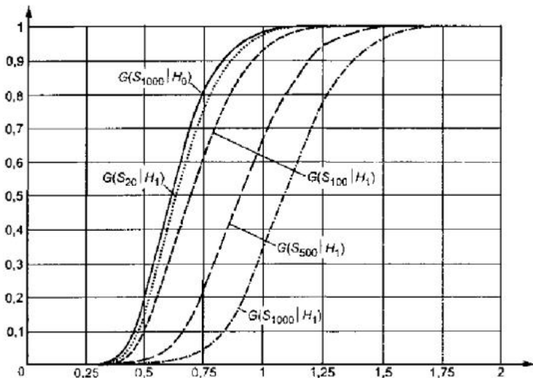
Рисунок 6 - Зависимость от n распределений G(S_n/2 | H_1) статистики S_K Колмогорова при сложной гипотезе ( H_0 - нормальное распределение, H_1 - логистическое, ОМП): n = 20, 100, 500, 1000
