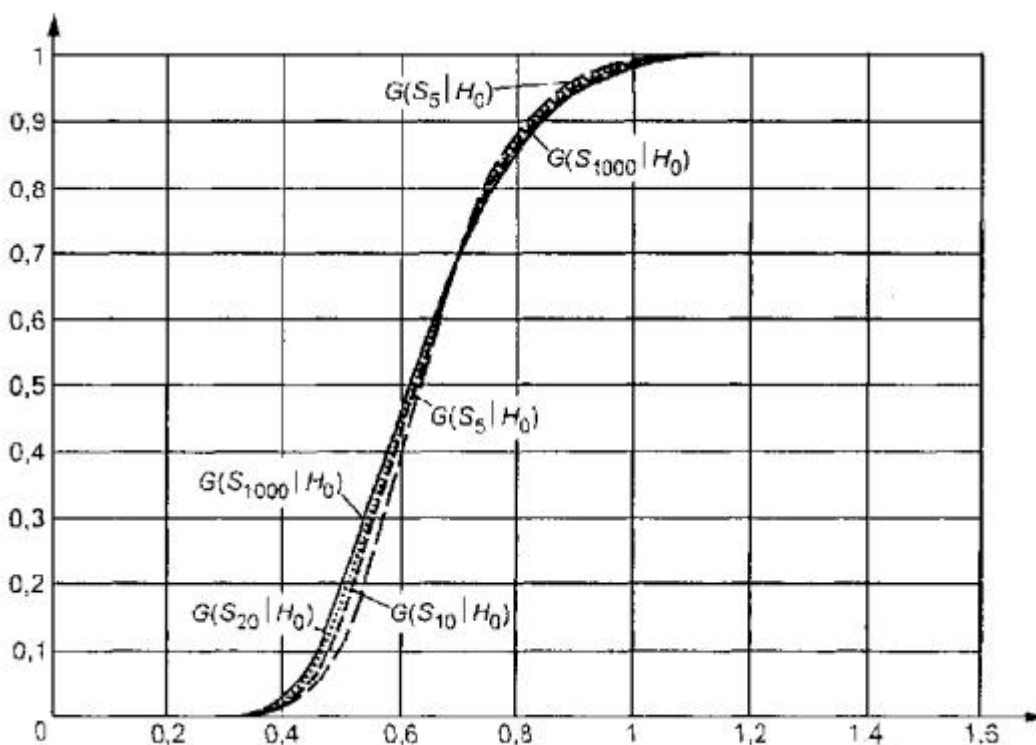
Рисунок 2 - Зависимость от n распределений G(S_n/2 H_0) статистики S_K Колмогорова при сложной гипотезе ( H_0 - нормальное распределение, ОМП): n = 5, 10, 20, 1000
