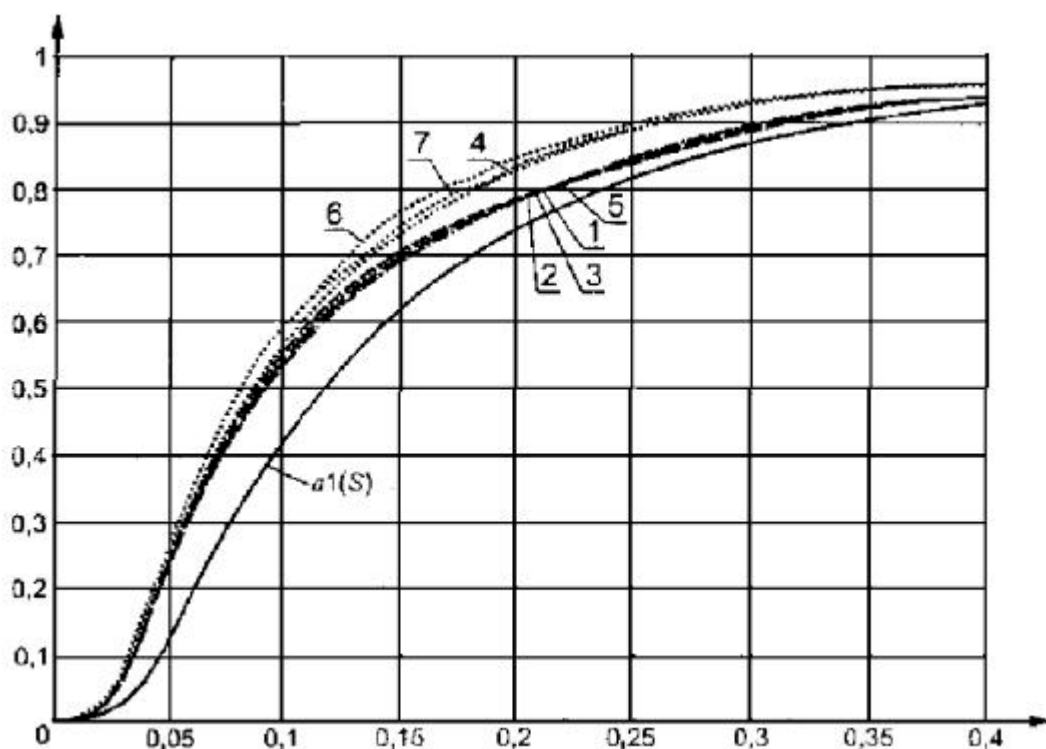
Рисунок 14 - Распределения G(S_n^{1/2}H_0) статистики S_0 Крамера - Мизеса - Смирнова при оценивании масштабного параметра закона, соответствующего гипотезе H_0 , (6 - максимального значения; 7 - Вейбулла, параметр формы), при использовании MD-оценок S_0
