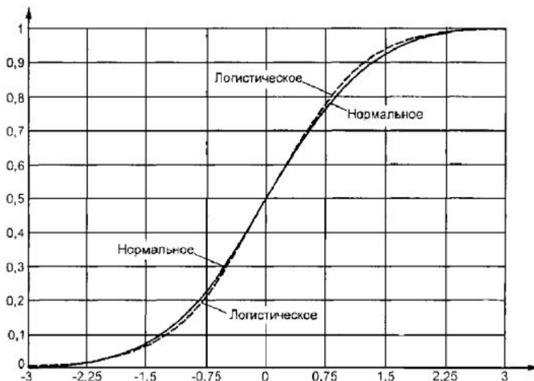
Рисунок 4 - Функции распределения нормального и логистического законов
