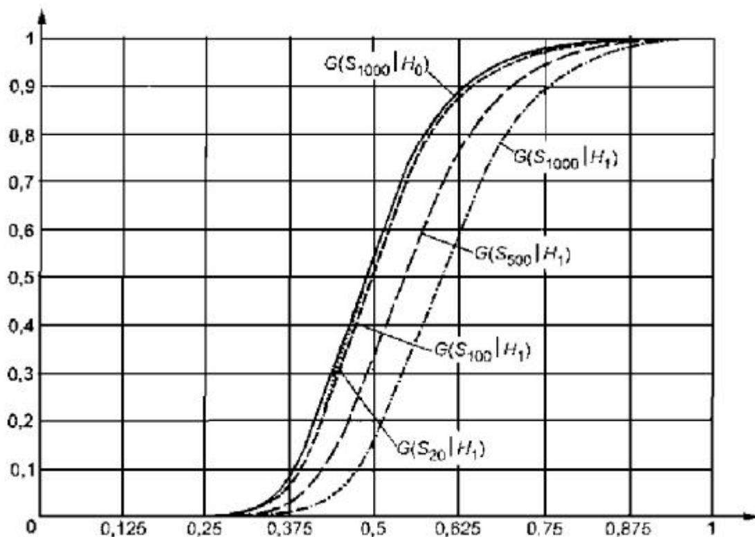
Рисунок 17 - Зависимость от n распределений G(S_n^{1/2}H_1) статистики S_K Колмогорова при сложной гипотезе ( H_0 - нормальное распределение; H_1 - логистическое; MD -оценки S_K ): n = 20, 100, 500, 1000
