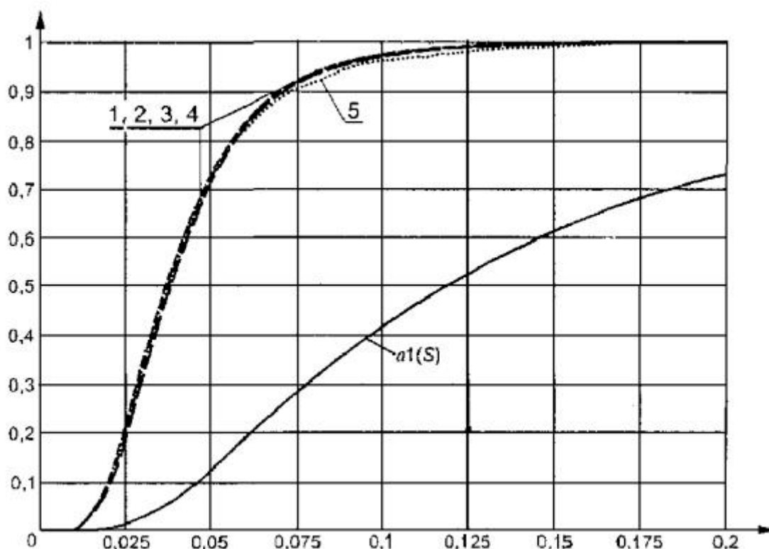
Рисунок 13 - Распределения G(S_n^{1/2}H_0) статистики S_\omega Крамера - Мизеса - Смирнова при оценивании двух параметров закона, соответствующего гипотезе H_0 , при MD -оценках S_\omega
