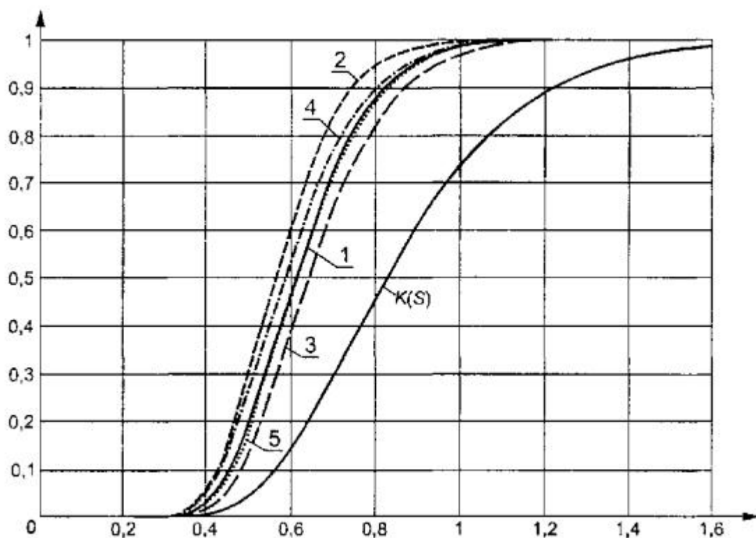
Рисунок 10 - Распределения G(S_n^{1/2}H_0) статистики Колмогорова S_K при оценивании двух параметров закона, соответствующего гипотезе H_0 (здесь и далее: 1 - нормального; 2 - логистического; 3 - Лапласа; 4 - наименьшего значения; 5 - Коши), при использовании ОМП. K(S) - функция распределения Колмогорова
