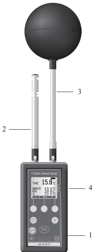
Рис.1 – Внешний вид прибора “ТКА-ПКМ”(24) 1 – БОИ; 2 – ИГ №1; 3 – ИГ №2 с черным шаром; 4 – Разъём связи с ПК.
