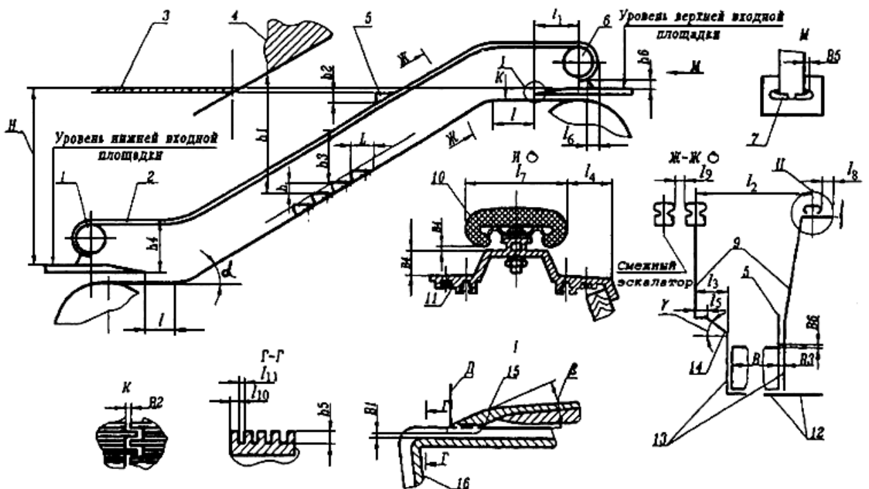
Рис.1. Схема устройства эскалятора:
